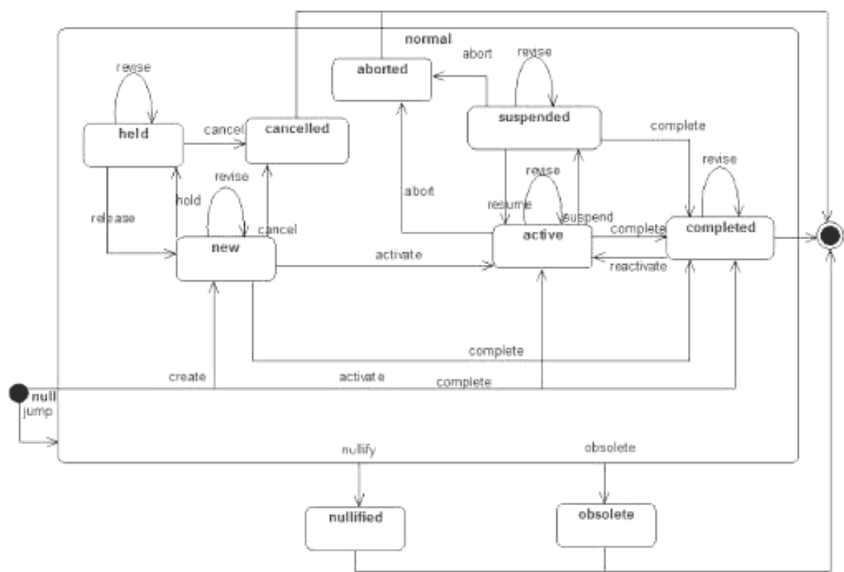
Рисунок 5 — Диаграмма перехода состояний класса Act (действие)
