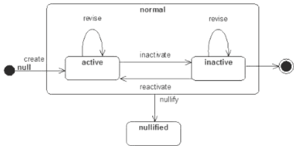
Рисунок 6 — Диаграмма перехода состояний класса Entity (сущность)
