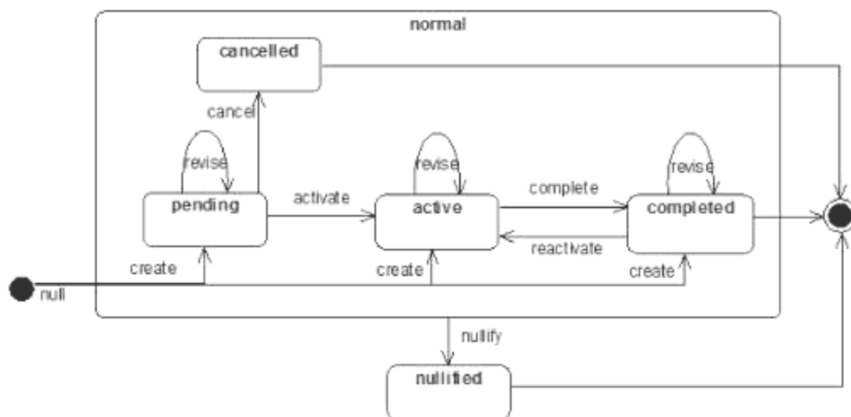
Рисунок 7 — Диаграмма перехода состояний класса ManagedParticipation (управляемое участие)
