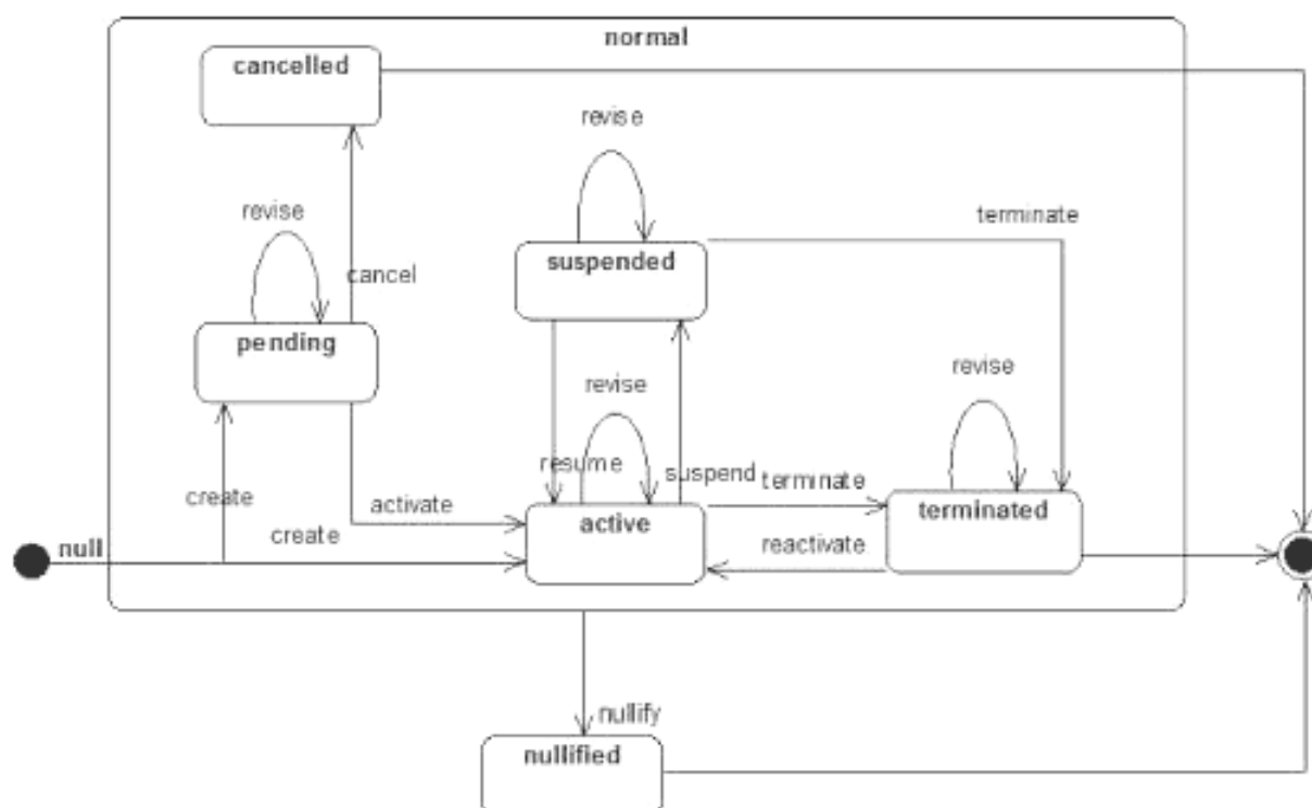
Рисунок 8 — Диаграмма перехода состояний класса Role (роль)
