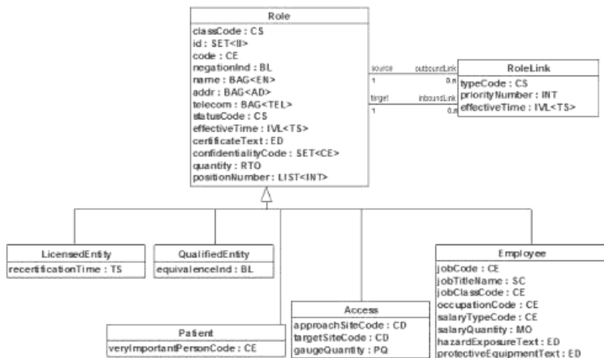
Рисунок 4 — Диаграмма классов предметной области Roles (роли)
