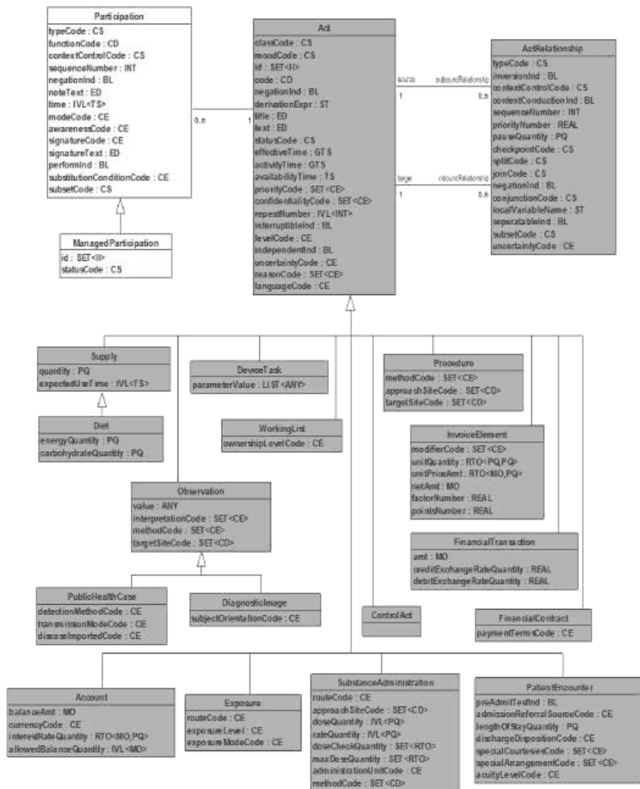
Рисунок 2 — Диаграмма классов предметной области Acts (действия)
