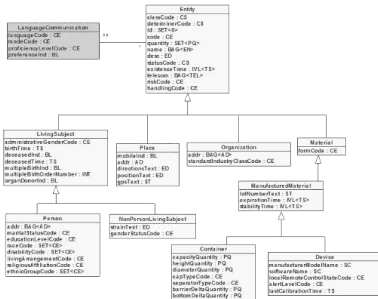
Рисунок 3 — Диаграмма классов предметной области Entities (сущности)
